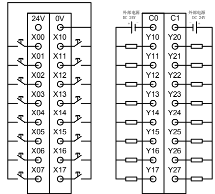
输入输出接线示意图
