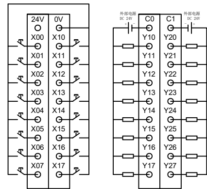
输入输出接线示意图
